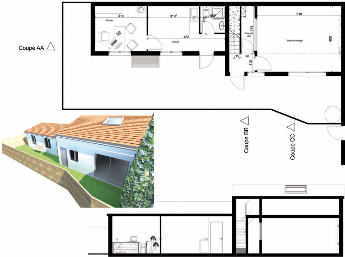
Coupe AA'
