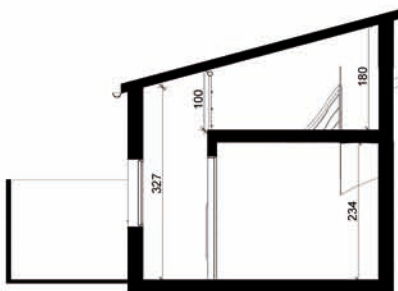
Coupe BB'
